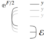
Lemma 2
