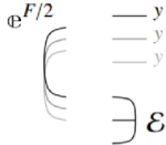
Lemma 2
