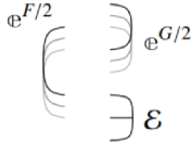
Lemma 1
